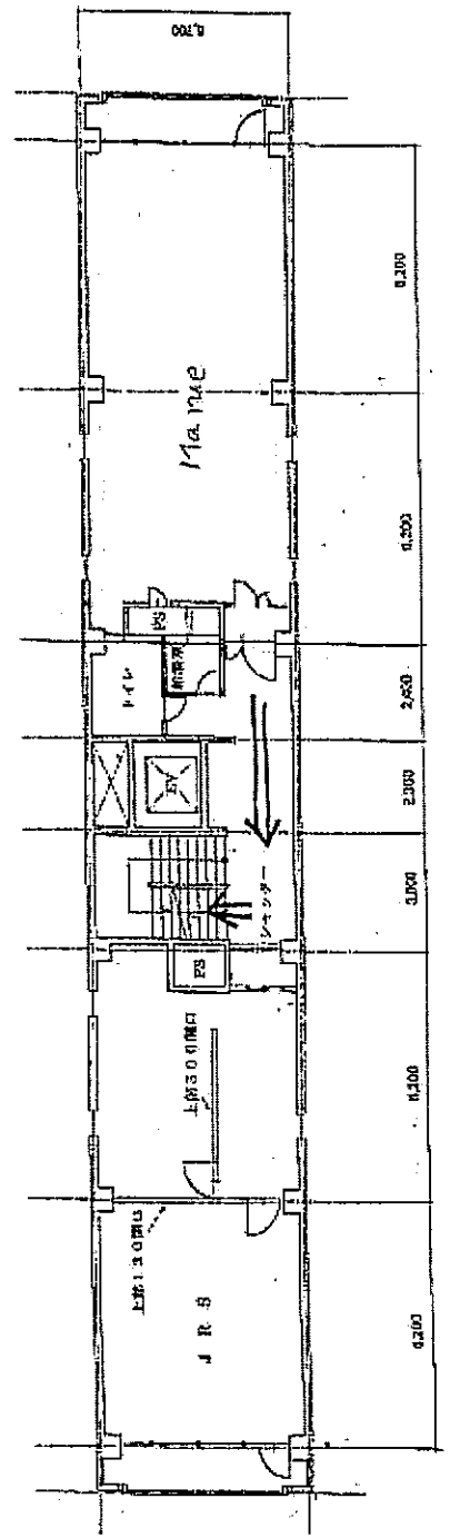
7階平面図 S-111100
